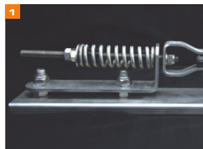
päätylukko: esi-koottu ja jatkuva jännitteinen.
