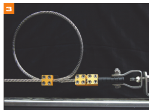
iskunvaimennin: esi-koottu vaijerin lenkki.
