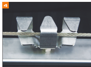
välikannake: ohitettava, tarvitaan jos vaijeria 15 m tai enemmän.
